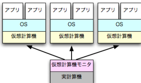
図? 仮想計算機によるサーバの集約(集約後)
