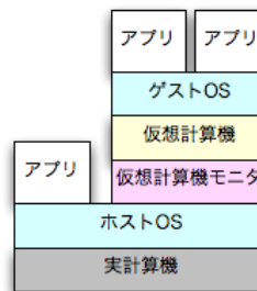
図? ホスト型仮想計算機モニタ
