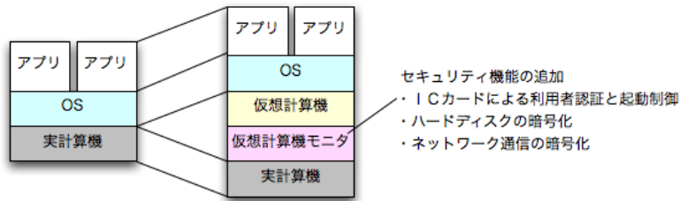
図? BitVisor の機能
